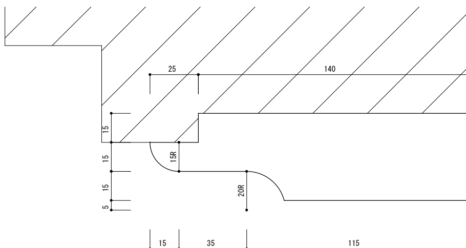
持ち送り置引き断面図 S=1/2
