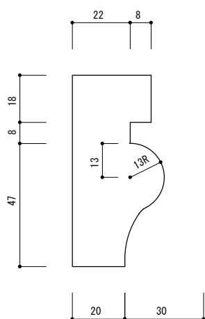
洗い出し現場引き断面図 S=1/2
