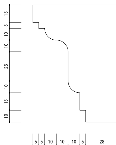
正面置引き断面図 S=1/2
