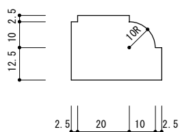
提灯置引き断面図 S=1/2
