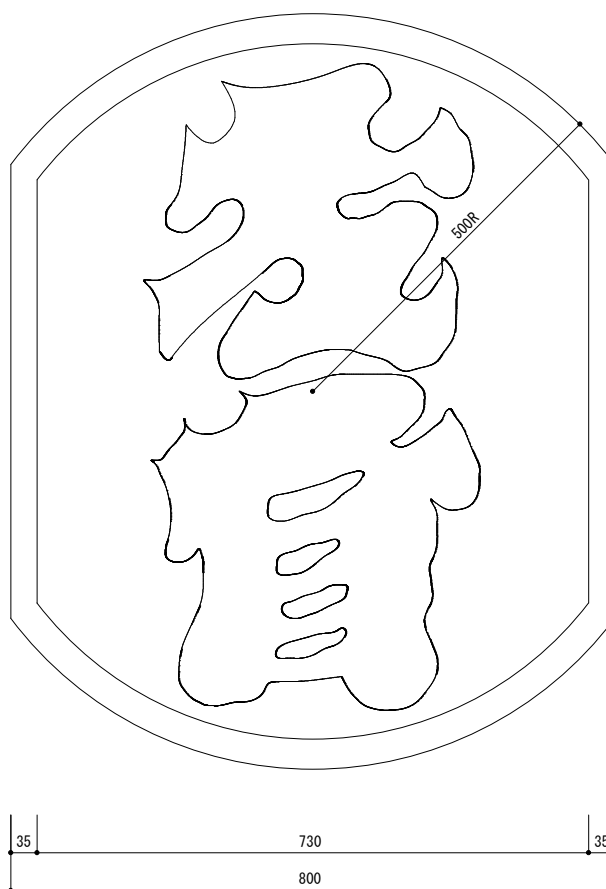
提灯置き寸法図 S=1/10
