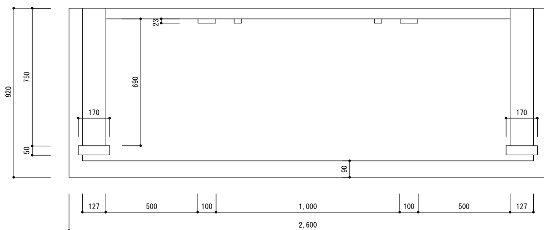
平面図 S=1/20
