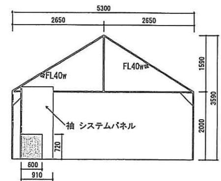
断面図
