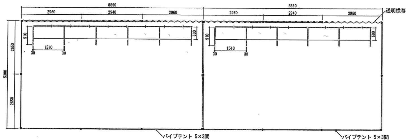
平面図
