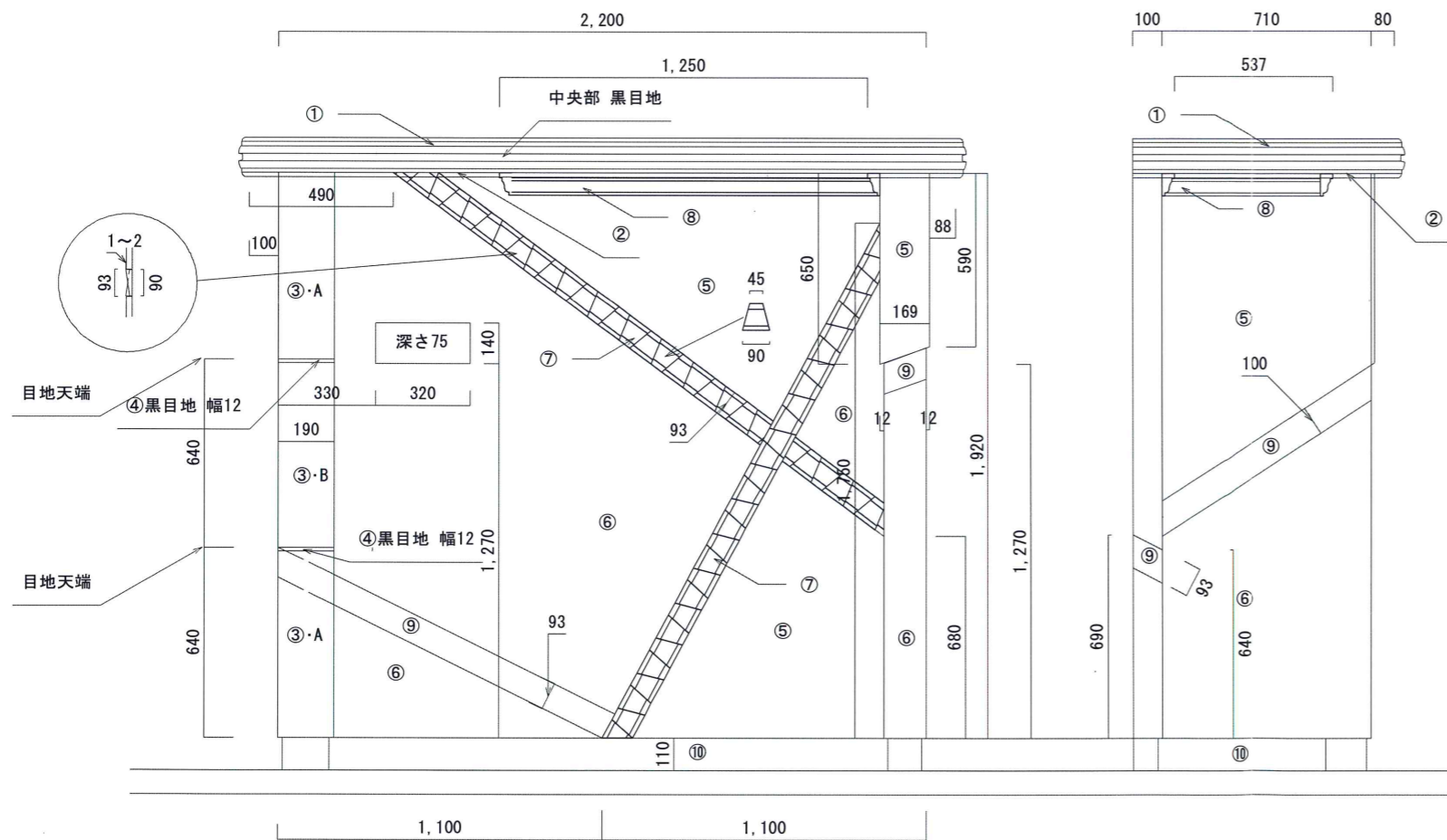
右袖壁内側図
