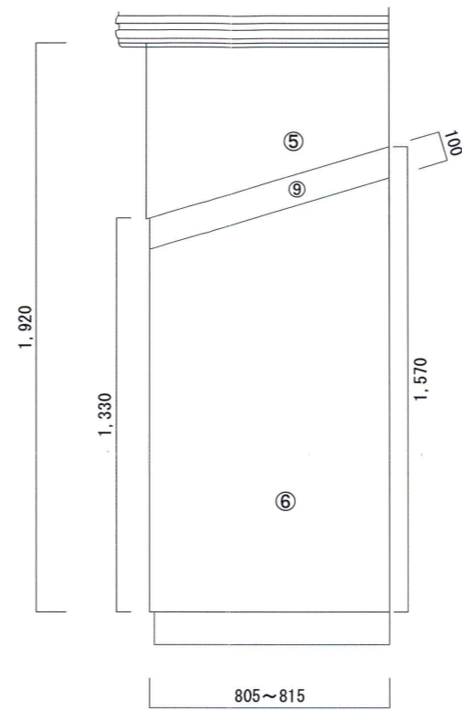
右袖壁外側図
