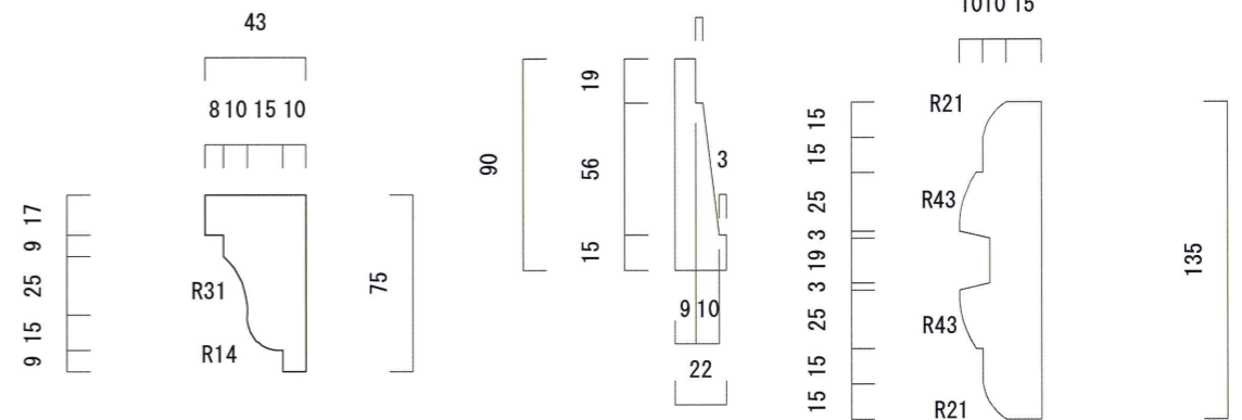
右袖壁外側図
