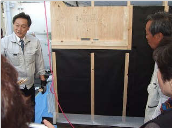
山中・林指導員による外壁モルタル通気工法
