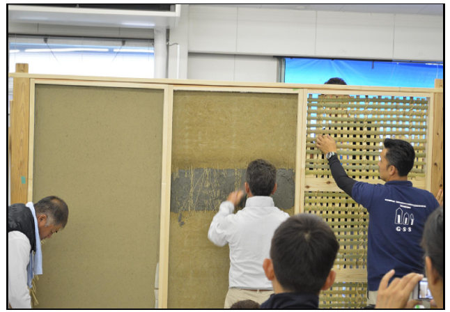
小舞壁の貫伏せ塗りを行う町田指導員
