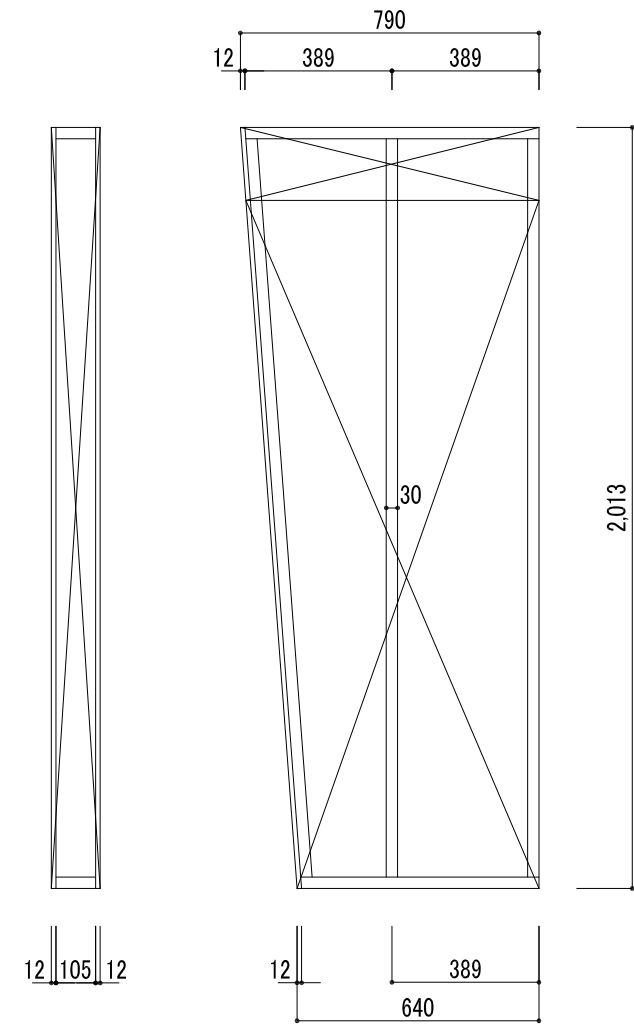
①下地図 S=1/20
