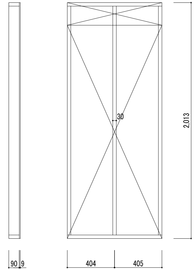
③下地図 S=1/20
