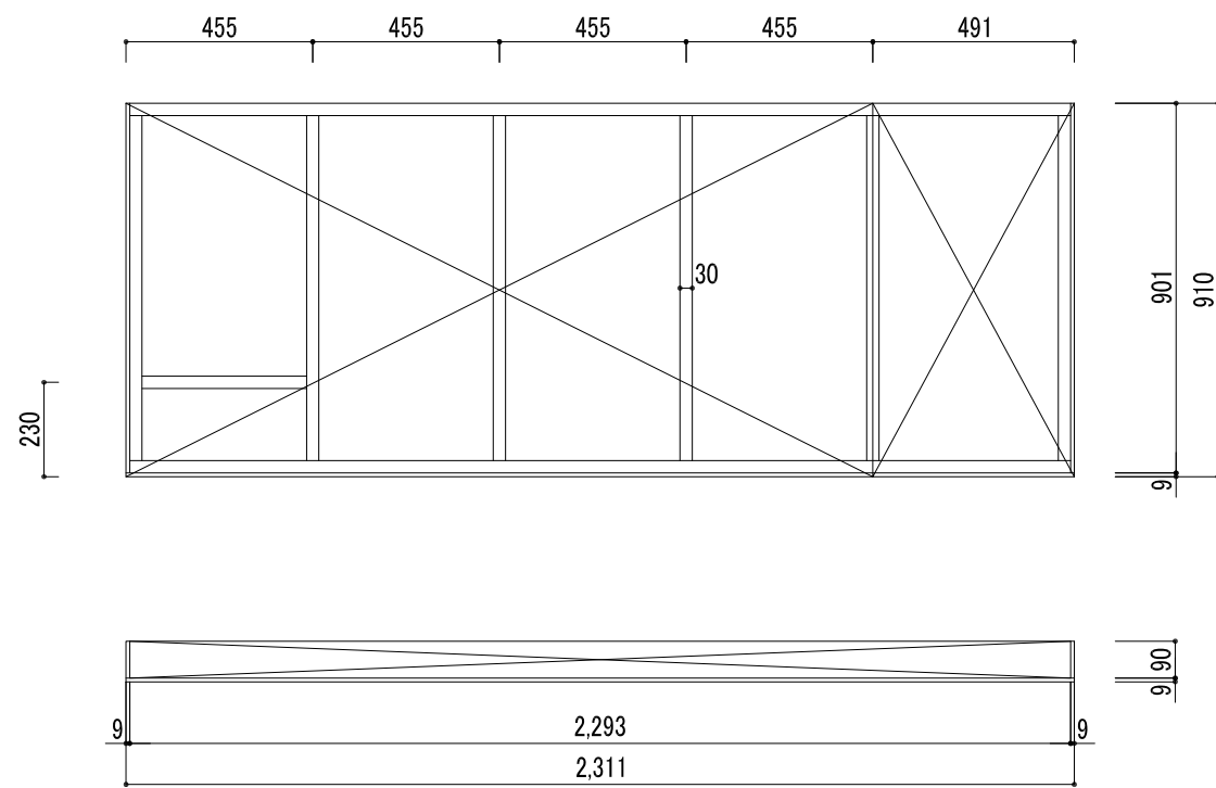
天井下地图 S=1/20
