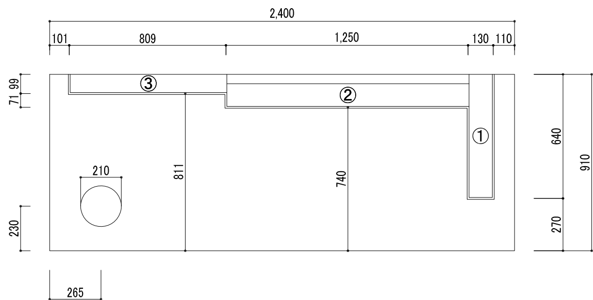
床下地图 S=1/20
