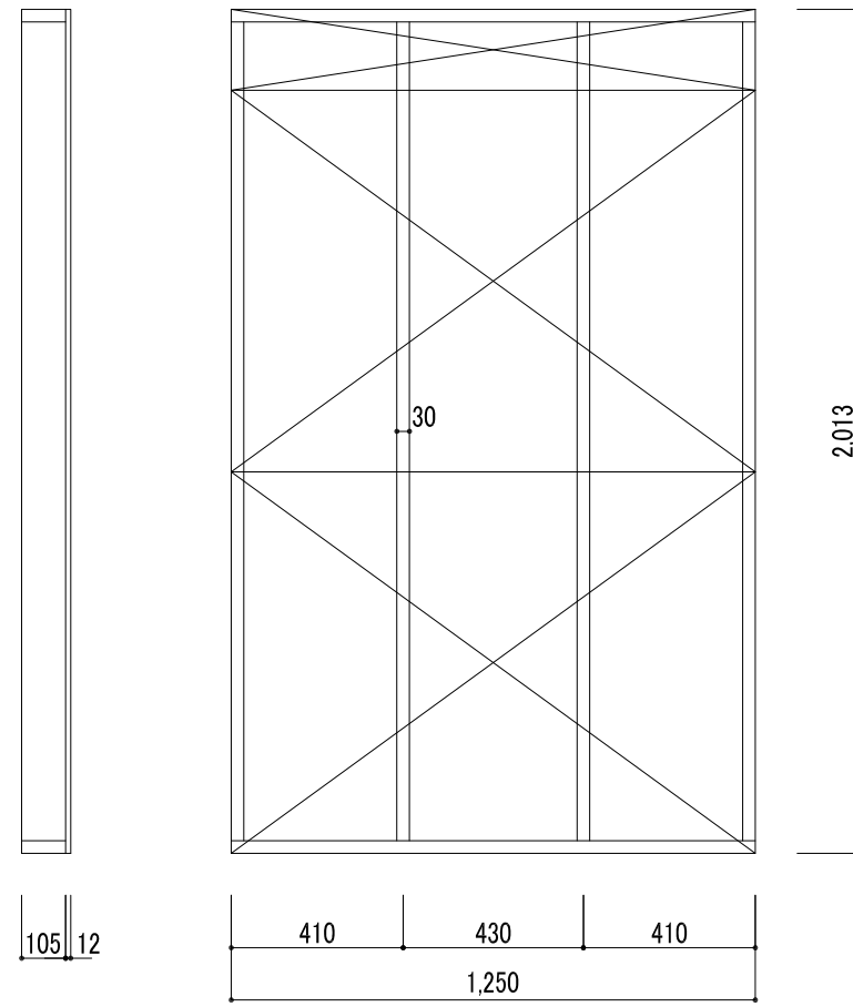
②下地図 S=1/20
