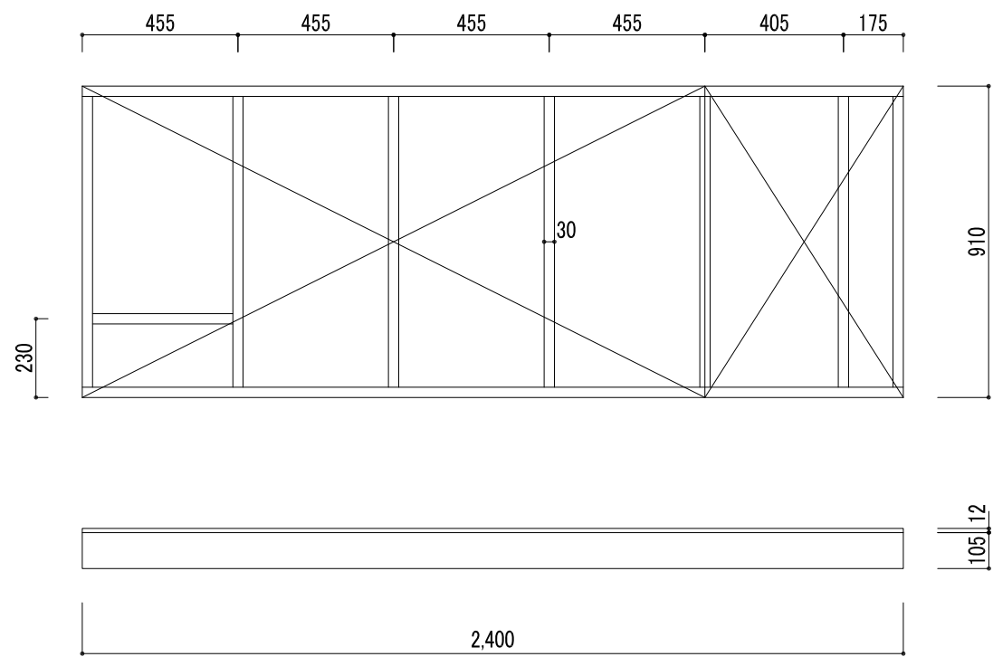
床下地图 S=1/20
