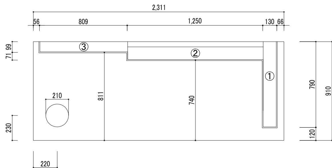
天井下地图 S=1/20
